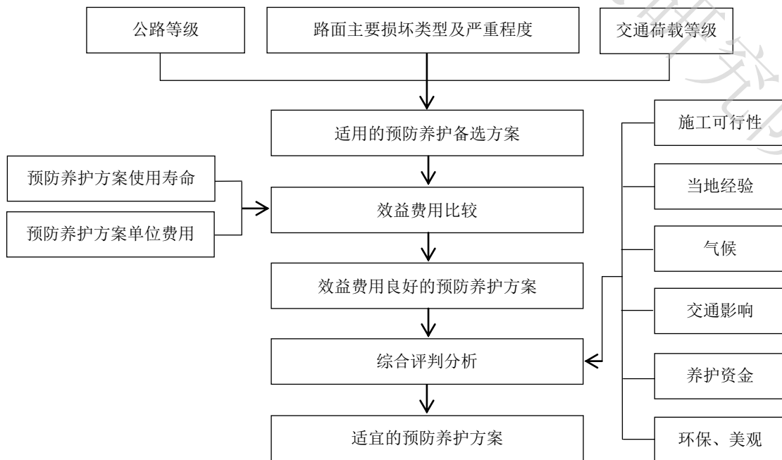
图 2 预防养护技术设计流程
