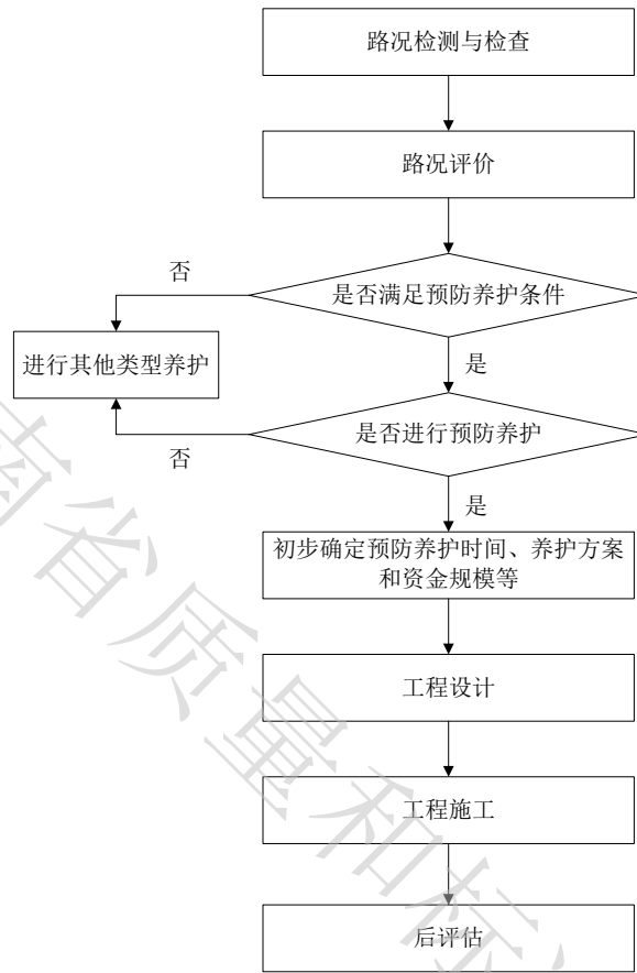
图 1 路面预防养护工作流程图
